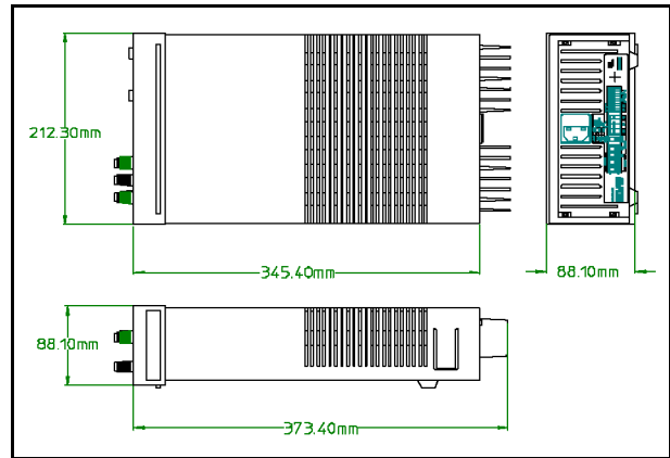
図 1. 外形図
