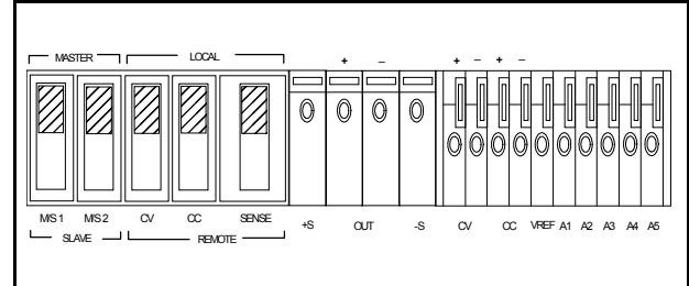
図 4. 電源投入チェックアウトのためのリア・パネル・コントロールのスイッチ設定
