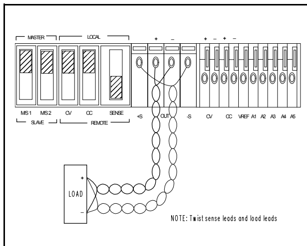
図5. リモート電圧検知
