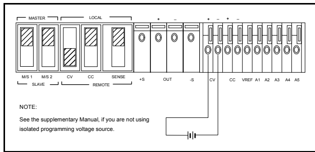
図 6. リモート電圧プログラミング、定電圧
