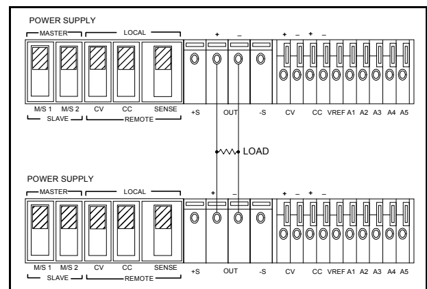
図 8. 2 台の装置の標準平行操作
